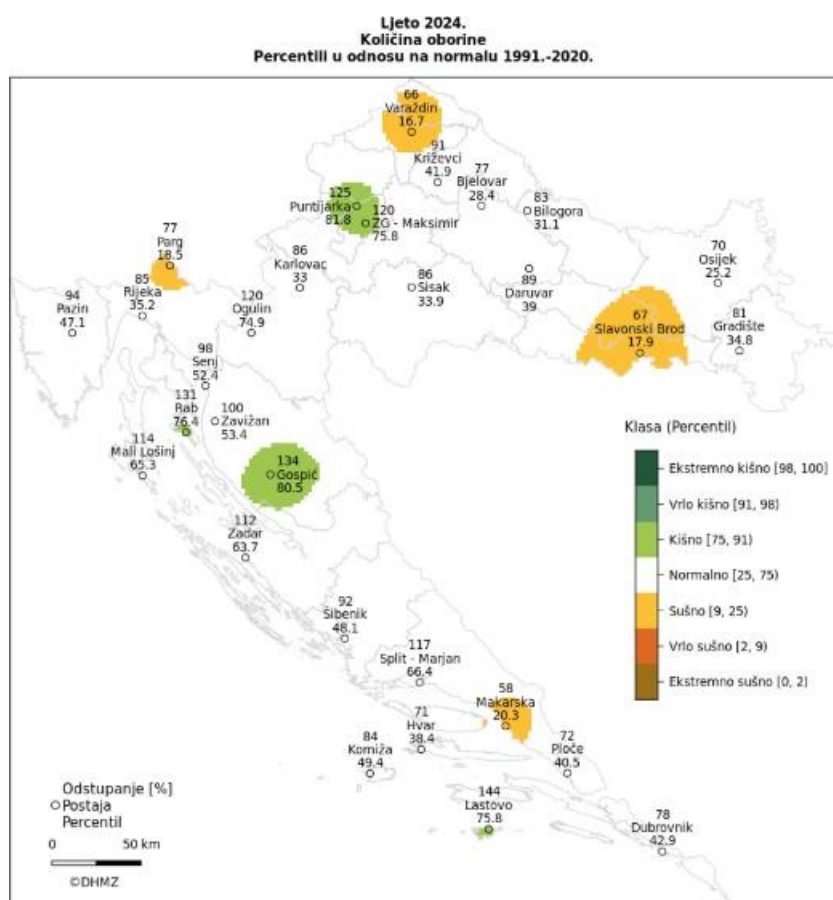
Slika 23: Odstupanje količine oborine u Hrvatskoj za ljeto 2024. godine
