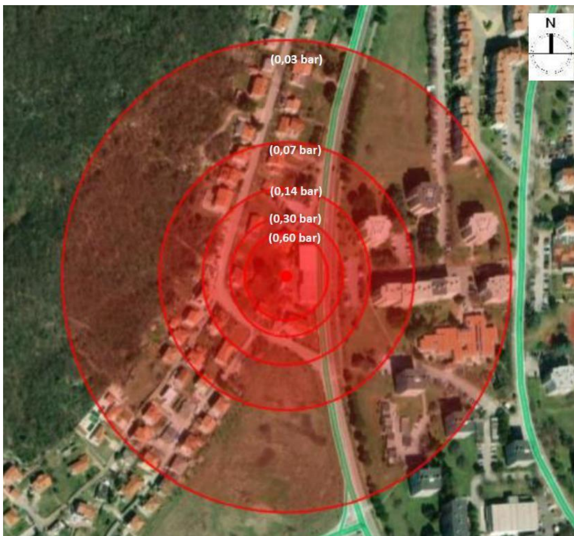
Slika 6. Zone ugroženosti eksplozije plinovite faze benzina
