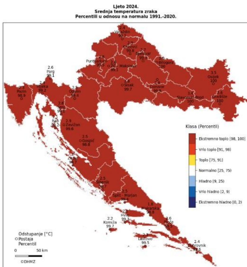
Slika 22: Odstupanje srednje mjesečne temperature zraka u Hrvatskoj za ljeto 2024. godine
